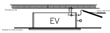
DETALHE DO PÓRTO DA UNIDADE EVAPORADORA TIPO CASSETE
