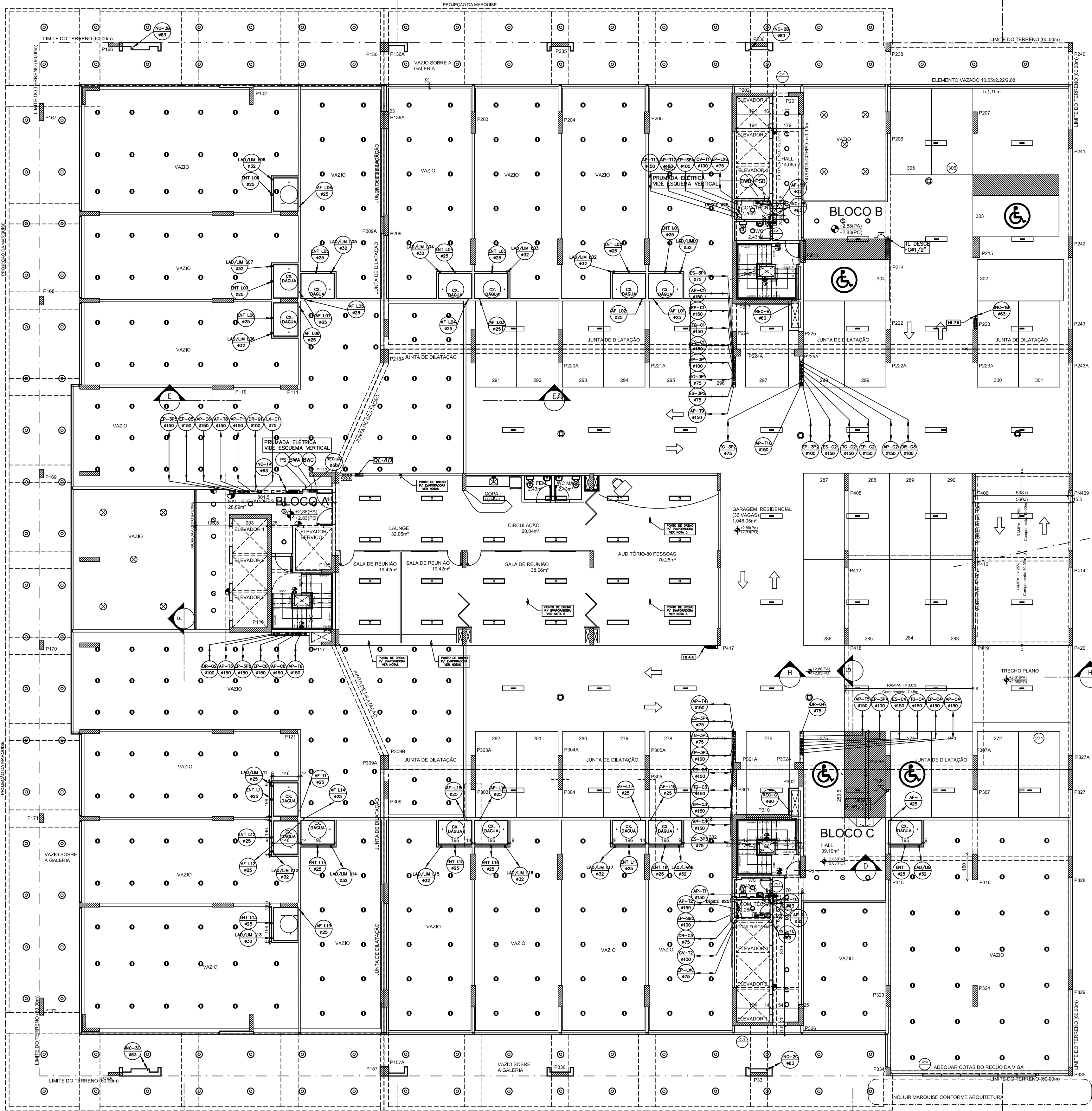
1 PLANTA BAIXA - SOBRELOJA ESC. 1/100
