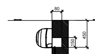
DETALHE DO PÓRTO DA UNIDADE EVAPORADORA TIPO HALL DETALHE DO CANAL METALIZADO INCRUSTADO NA PAREDE O TIPO CILINDRO PARALELO
