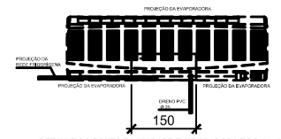
DETALHE DO PÓRTO DA UNIDADE EVAPORADORA TIPO HALL
